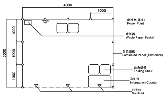
俯视图 (4.0mL x 3.0mW x 2.5mH)
