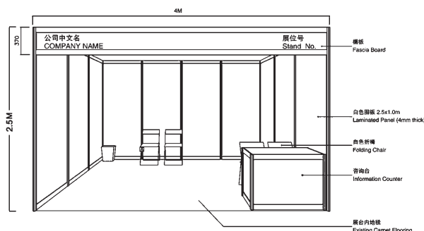
前视图 (4.0mL x 3.0mW x 2.5mH)
